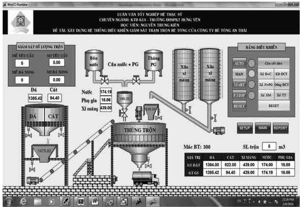
Hình 3b. Giao diện điều khiển giám sát trộn bê tông tự động
