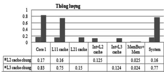
Hình 4e. Giá trị trung bình của thông lượng ở các nút của CMP 4 nhân/10 luồng với L2 cache chung và L3 cache chung
