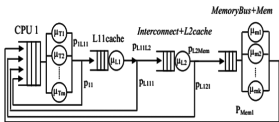
Hình 2. MCPFCQN rút gọn cho CMP đa luồng có 2 cấp cache với L2 cache chung
