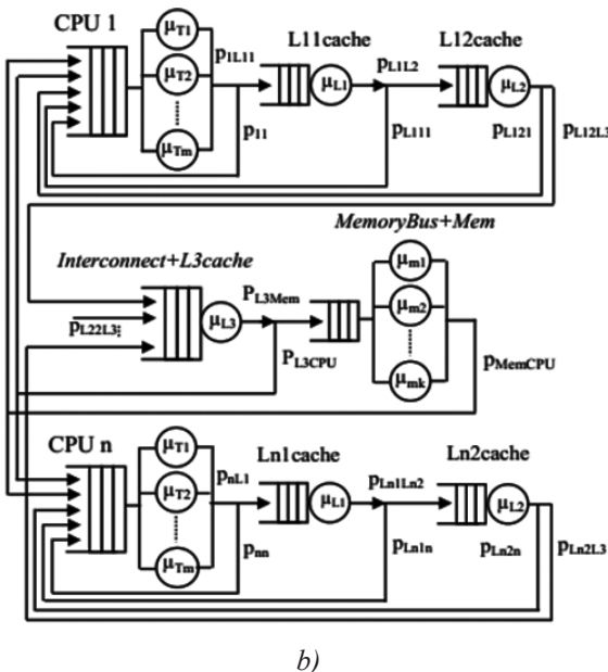
Hình 1. Mô hình MCPFCQN cho CMP đa luồng n nhân
