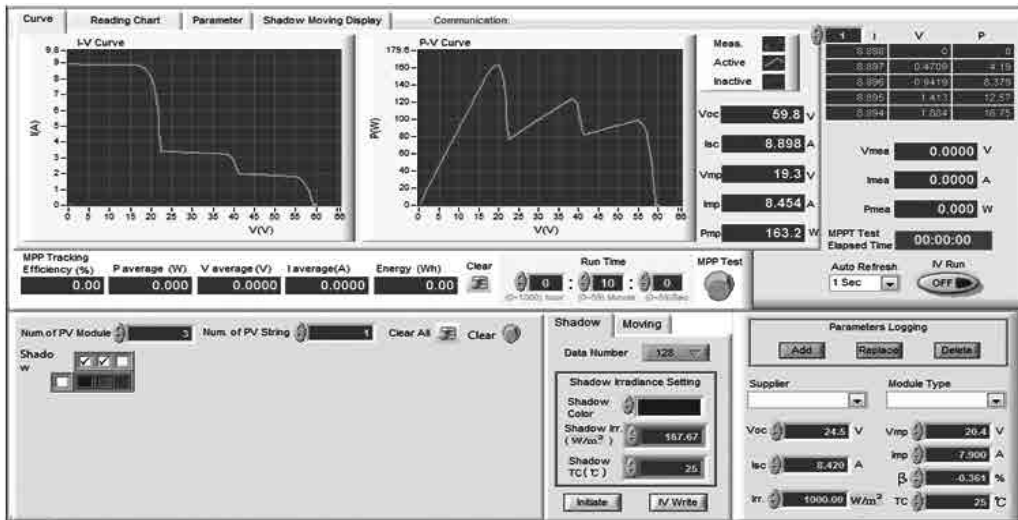
Hình 6. Giao diện thiết lập thông số dàn Pin PV khi bị che chắn 2 phần, cường độ ánh sáng S_1 = 167.67 \text{ W/m}^2 và S_2 = 320.00 \text{ W/m}^2 , nhiệt độ môi trường T = 25^\circ\text{C}
