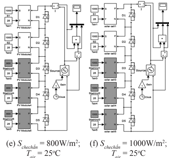
Hình 2. Mô hình mô phỏng của dàn Pin PV mắc nối tiếp khi thay đổi S_{chech\hat{a}n} nhiệt độ không đổi
