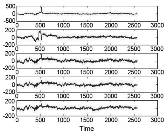
Hình 4. Dữ liệu điện não đồ 5 kênh
