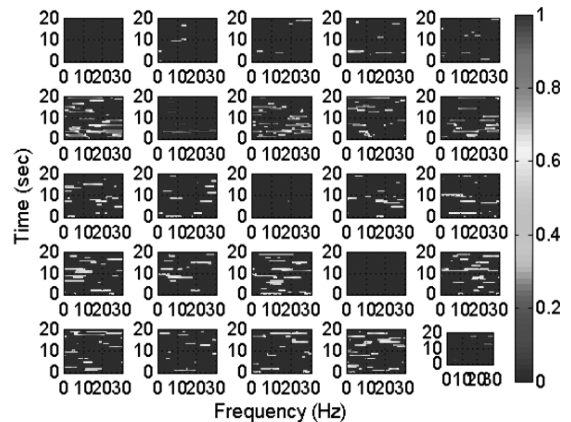
Hình 5. Sự phụ thuộc theo thời gian của 5 kênh dữ liệu điện não đồ
