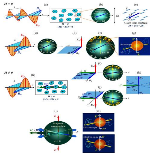
Hình 5: Mô hình giải thích tương tác magnon-plasmon [15].
