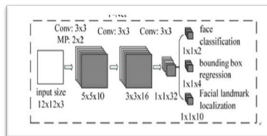
Hình 3: Mạng P-Net
