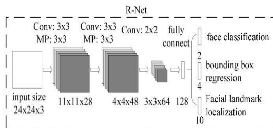
Hình 4: Mạng R-Net
