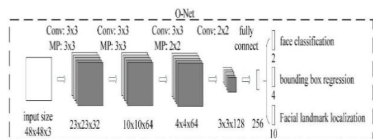
Hình 5: Mạng O-Net
