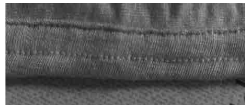
Hình 6. Đường may với mật độ 6 mũi/1cm
