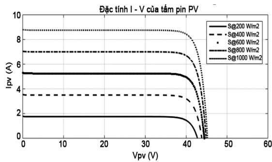
Hình 4. Đặc tuyến I-V của mô đun PV khi T = 25^{\circ}\text{C} và S thay đổi
