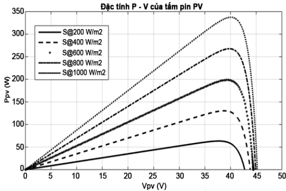
Hình 3. Đặc tuyến P-V của mô đun PV khi T = 25^{\circ}\text{C} và S thay đổi
