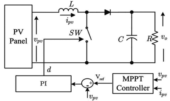
Hình 6. Sơ đồ mạch điện của hệ thống PV
